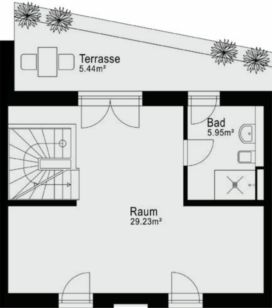
2. OG
